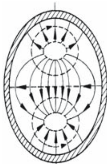
Abb. 3.2 Elektrische Feldverteilung einer TM1-Resonatorwelle in einem Ellipsoid. Der Vergleich mit Abb. 3.1 bestätigt, dass die Ausmusterung der mitotischen Figuren exakt nach der Kraftverteilung der Hohlraumresonatorwelle verläuft. Der dynamische Verlauf der mitotischen Teilung lässt sich als Überlagerung passender Hohlraumresonatorwellen (s. Tab. 3.1) verstehen (aus [39]).
